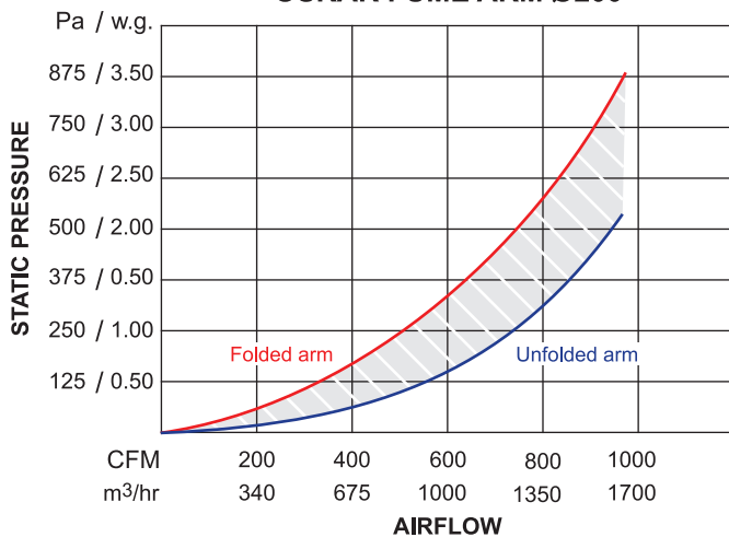
OSKAR FUME ARM Ø200
