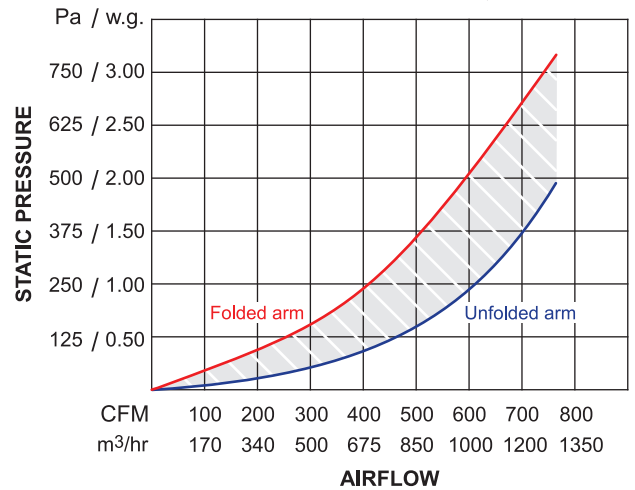
OSKAR FUME ARM Ø160
