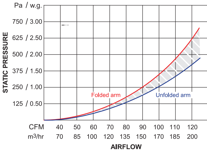
OSKAR FUME ARM Ø75
