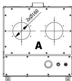
Podwójny wlot
