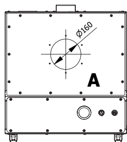
Pojedynczy wlot
